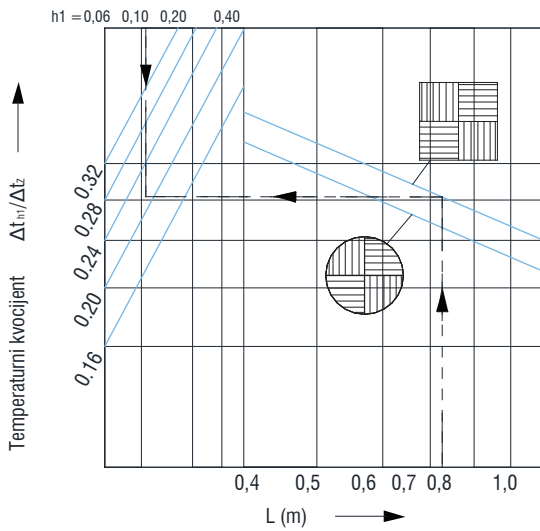
Temperaturni kvocijent SDV-K stubno
