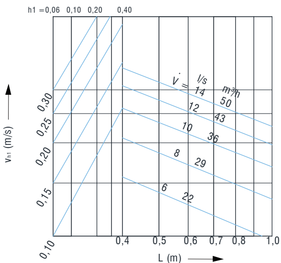
Razina zvučne snage i pad tlaka SDV-KO-T
