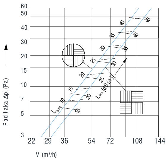
Razina zvučne snage i pad tlaka SDV-T
