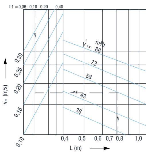
Razina zvučne snage i pad tlaka SDV-KK-K stubno
