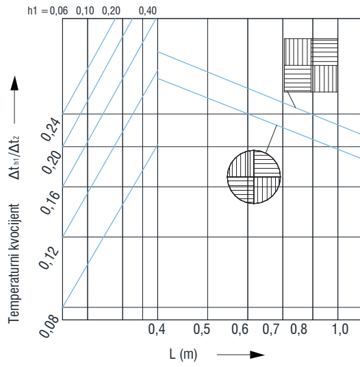
Temperaturni kvocijent SDV-T stubno
