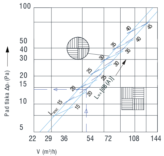
Razina zvučne snage i pad tlaka SDV-K
