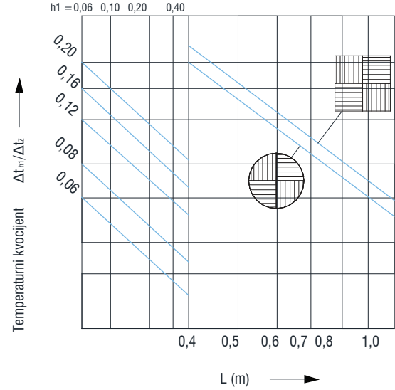
Temperaturni kvocijent SDV-T podno
