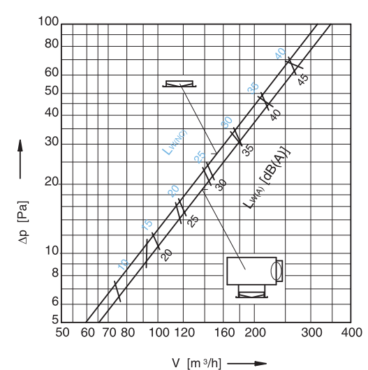
Dijagram razine buke i pada tlaka DK 200
