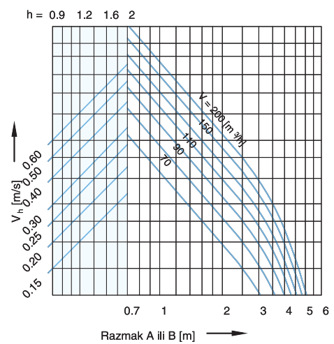
Kvadratni difuzor - DK 160
