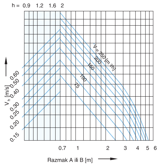
Kvadratni difuzor - DK 200
