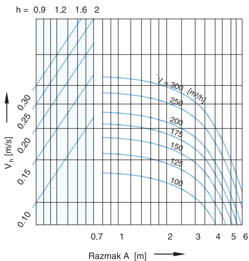
Raspored difuzora - DK 250 (u više od jednog reda, ako je B = 2,80 m)
