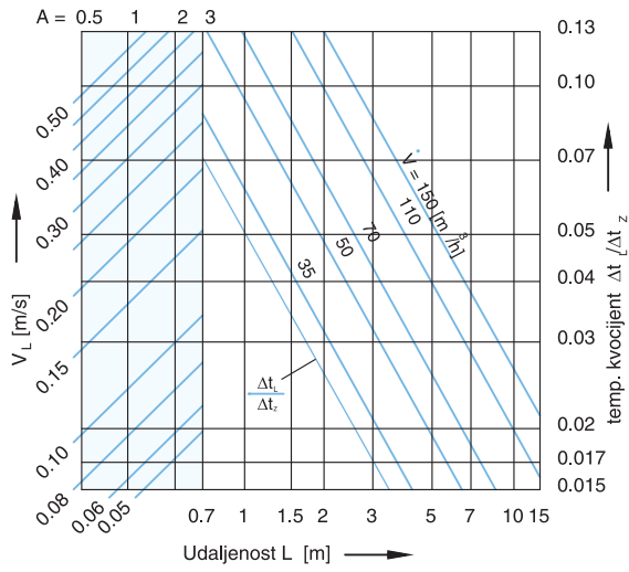
Raspored difuzora - DK 160 (u više od jednog reda, ako je B = 2,80 m)
