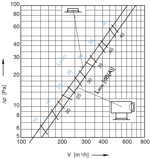
Dijagram razine buke i pada tlaka DK 315 - I
