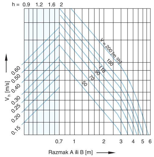
Raspored difuzora - DK 160 (u jednom ili više redova, ako je B ≥ 4,00 m)
