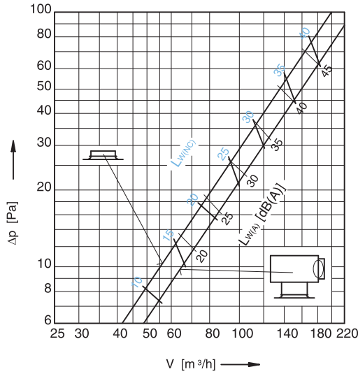
Dijagram razine buke i pada tlaka DK - I 160
