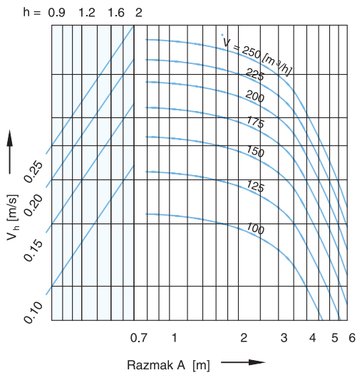
Brzina zraka uz zid - DK 200
