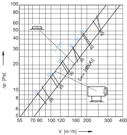
Dijagram razine buke i pada tlaka DK 200 - I
