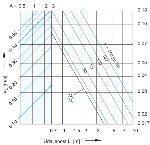
Brzina zraka uz zid - DK 160
