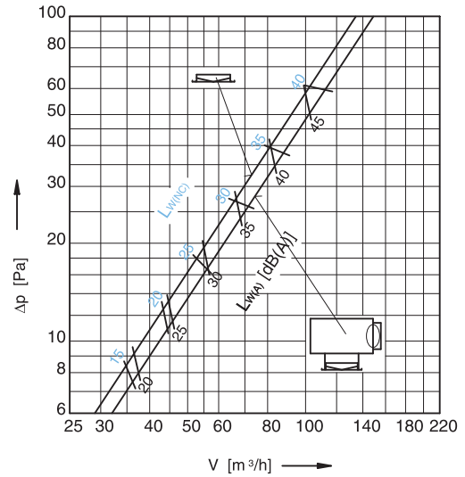
Dijagram razine buke i pada tlaka DK 160
