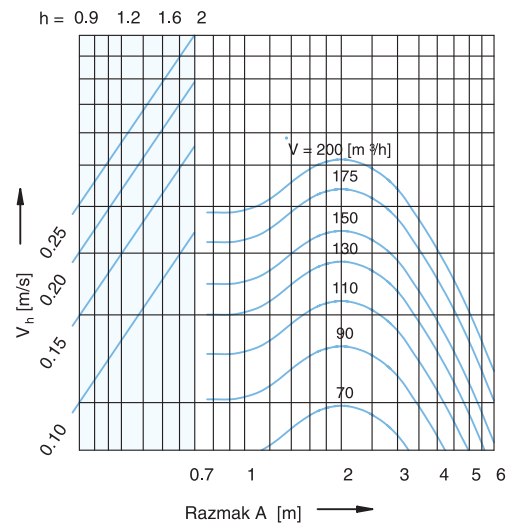
Raspored difuzora - DK 125 (u jednom ili više redova, ako je B ≥ 4,00 m)
