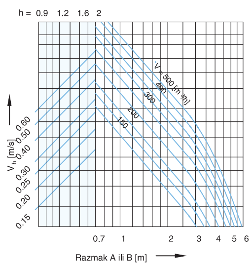
Kvadratni difuzor - DK 315
