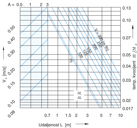
Brzina zraka uz zid - DK 200
