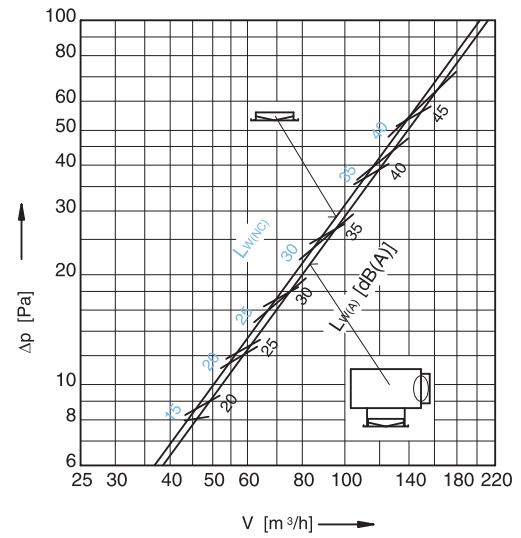
Dijagram razine buke i pada tlaka DK 200
