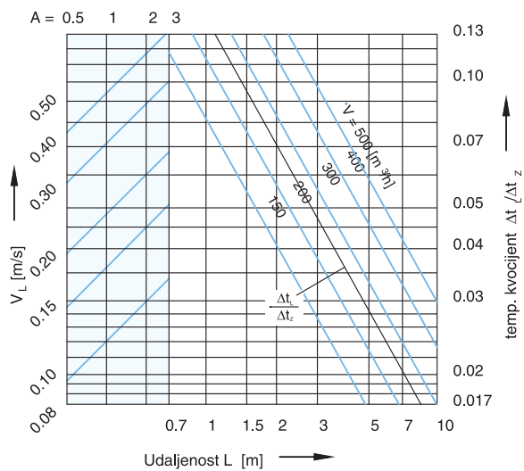
Brzina zraka uz zid - DK 315
