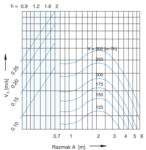
Raspored difuzora - DK 250 (u jednom ili više redova, ako je B ≥ 4,00 m)
